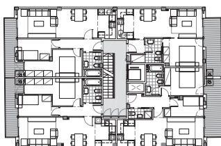
PLANTES 1 i 2 E 1:500
