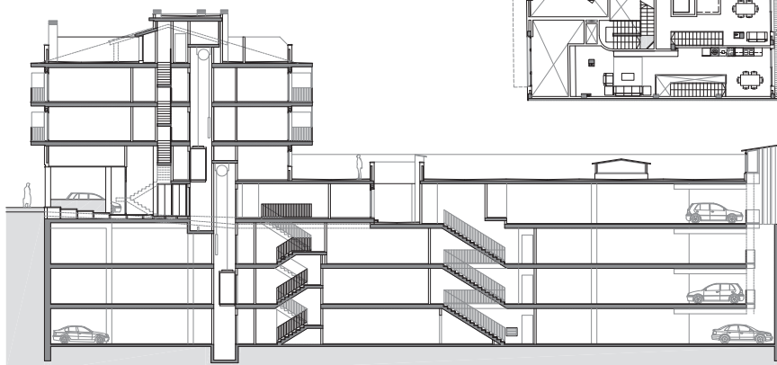
SECCIÓ E 1:500
