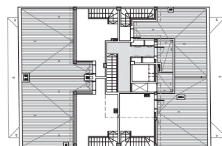
PLANTA coberta E 1:500
