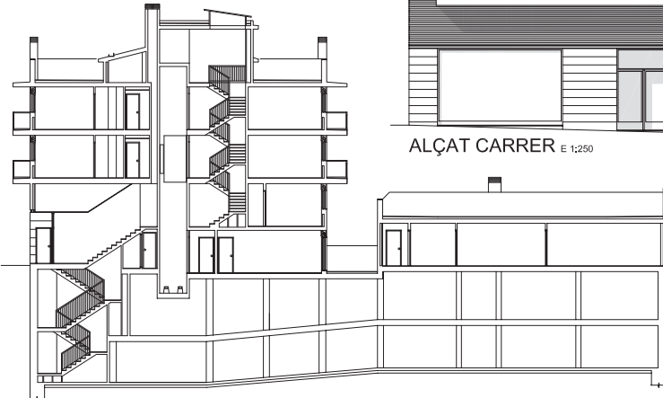
SECCIÓ E 1:400
