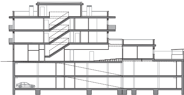
SECCIÓ E 1:500
