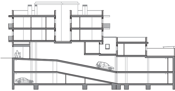
SECCIÓ E 1:500
